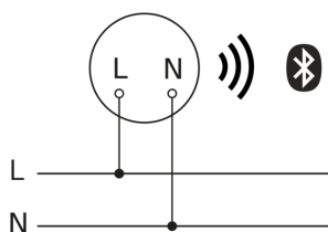
Diagrama electrónico interconexión esclavo maestro de radio
